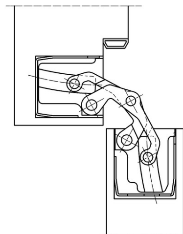
Marco macizo 90°
