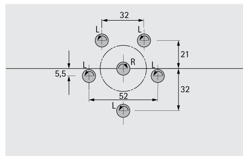
Esquema de perforaciones
