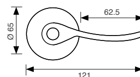
Esquema
